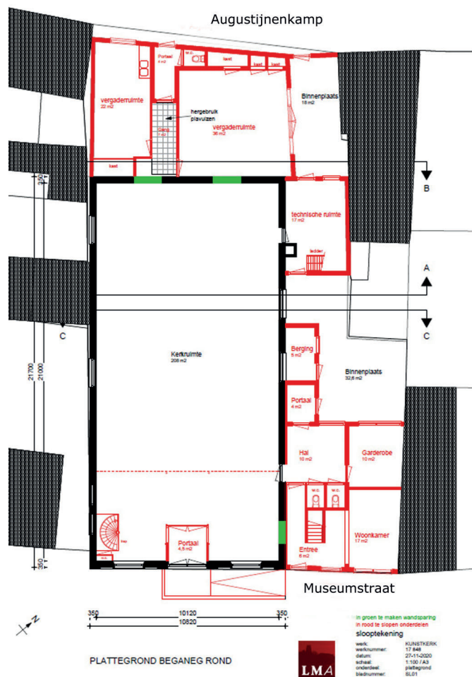
Afb. 3. De locaties van de drie te slopen bouwdelen binnen het plangebied. Dit zijn de drie onderzoekslocaties (sloop- en bouwplan door Lugten Malschaert Architecten bv, d.d. 10-2-2021, werknummer 17 848, bladnummer BN-01).
