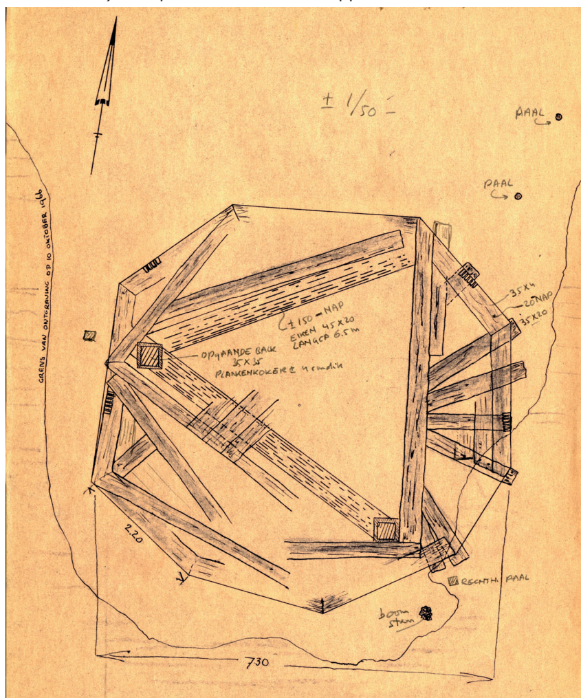
Afb. 11. De tekening van de fundering van de stadsgalg, (vermoedelijk) getekend door dhr. Bokma, zoals waargenomen op 10 oktober 1966.
