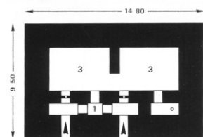
502, Doppelgruppenunterstand Gebouwd: 121; resteert: 59. Ontwerp vrijgegeven: 1939 Beton: 629 m 3
