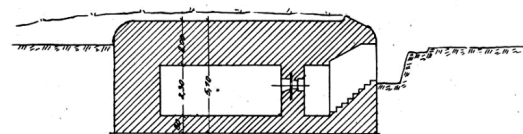
schnitt A-B
