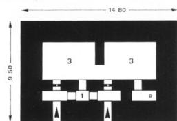
502, Doppelgruppenunterstand Gebouwd: 121; resteert: 59. Ontwerp vrijgegeven: 1939 Beton: 629 m³
