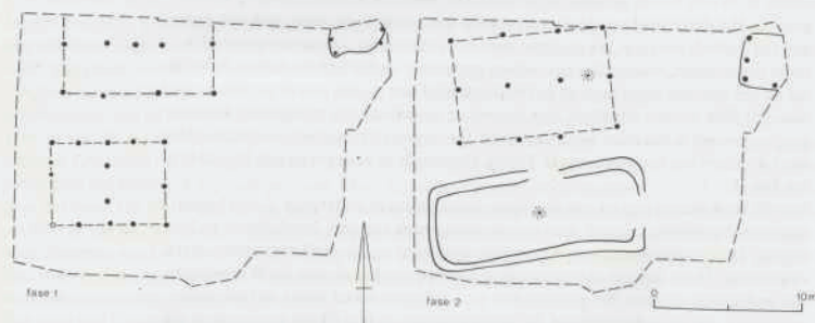
Afb. 12. *s-Gravenhage: Johan van Oldenbarneveltdaan. Huisplattegronden en hutkommen uit de 7e eeuw. Tek. J. T. de Jong.
