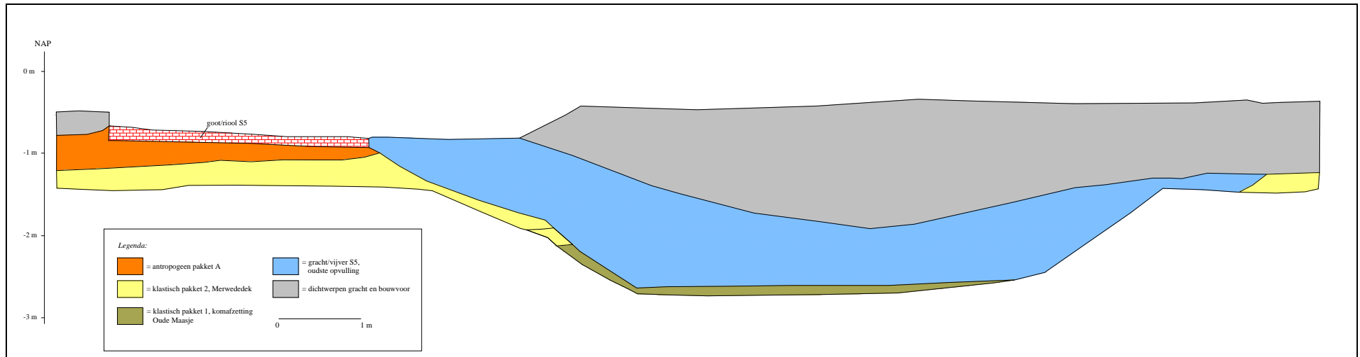
Afb. 8. Dwarsdoorsnede (zuidprofiel sleuf 1) van de gracht/vijver S5 met het riooltje S2 dat daarop uitkwam.
