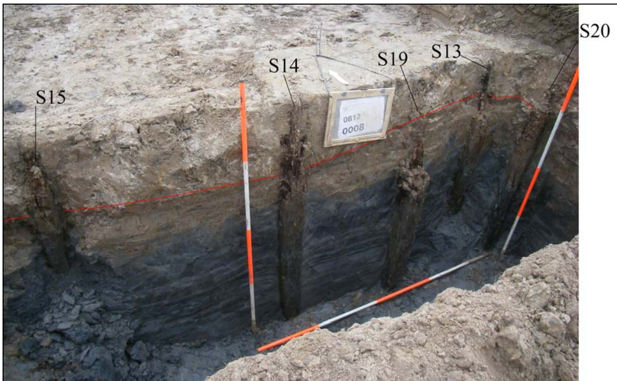
Afb. 11. Foto van een aantal van de funderingspalen van de noordgevel van het herenhuis. De rode lijn is de grens tussen het ophogingspakket en de natuurlijke ondergrond. (Fotorichting noordoost).
