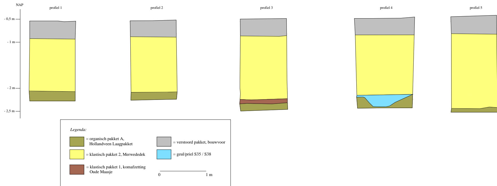
Afb. 16. Geïnterpreteerd lithostratigrafisch bodemprofiel van sleuf 7 op basis van de profielkolommen. Voor de locaties van de profielkolommen zie afb. 15.
