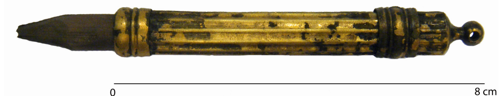
Afb. 36. Grafiethouder van messing. Voorin is de nog aanwezige en in een punt geslepen staaf grafiet te zien.
